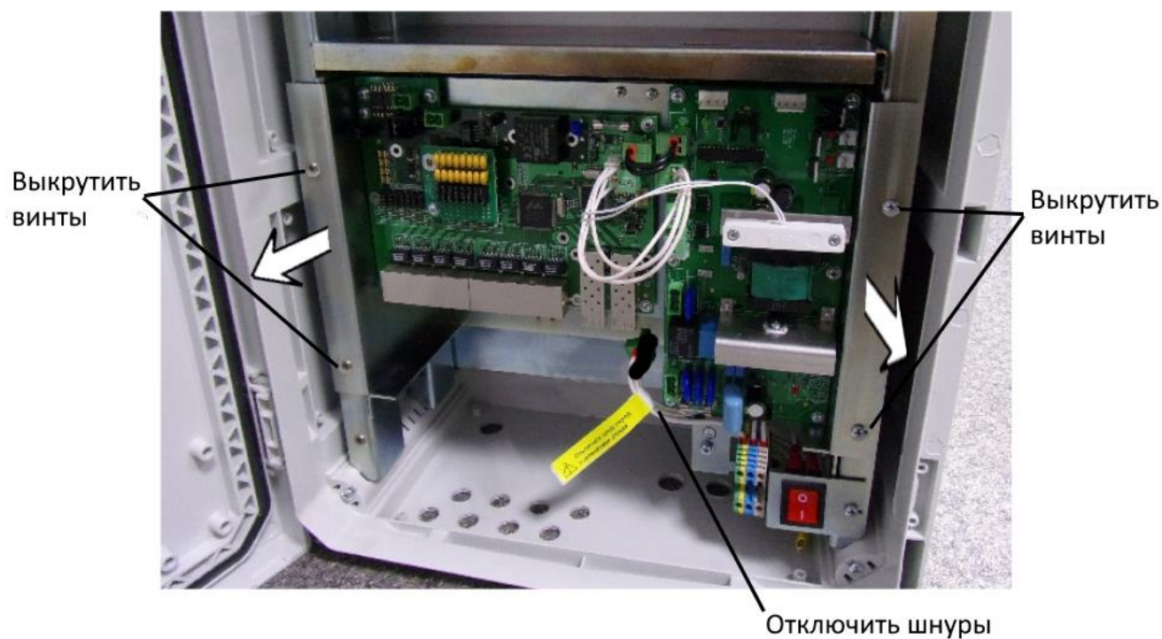
Рис. 7.1.2. Извлечение электронного узла
