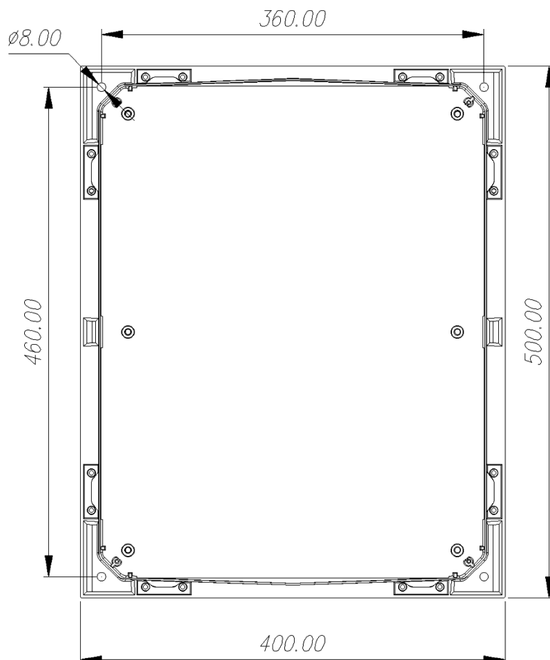
Рисунок 7.2 - Разметка крепления
