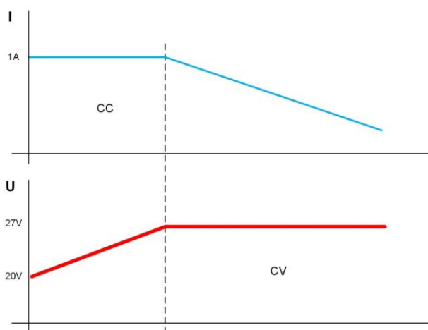
Рисунок 3.11.2 – Зависимость постоянного тока и напряжения заряда АКБ.
