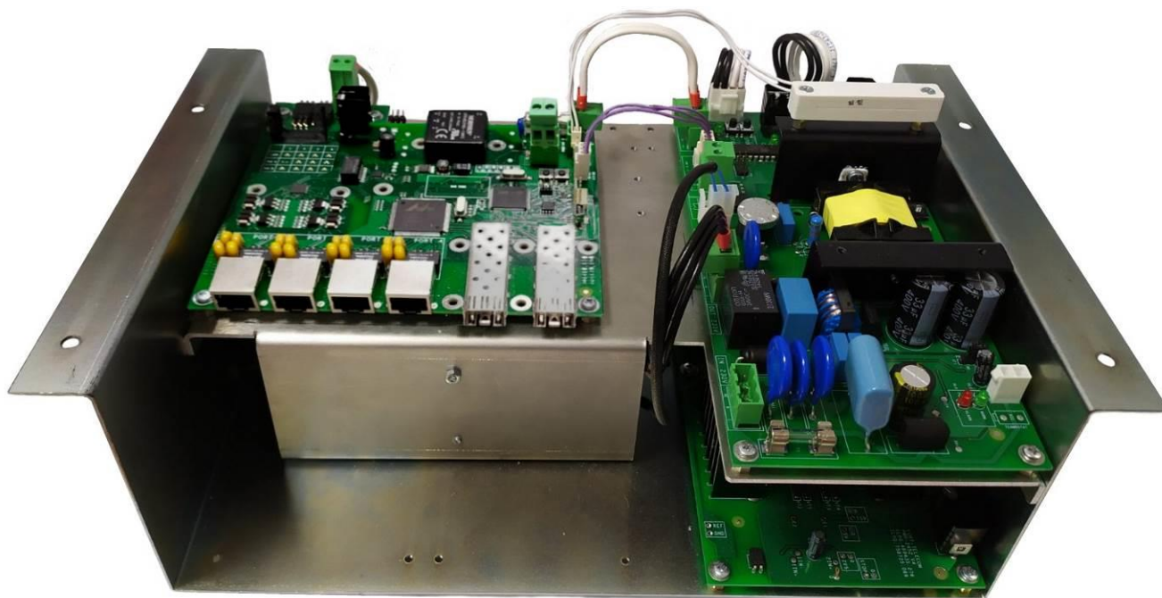
Рисунок 3.4.1 - Платы коммутатора и блоков питания
