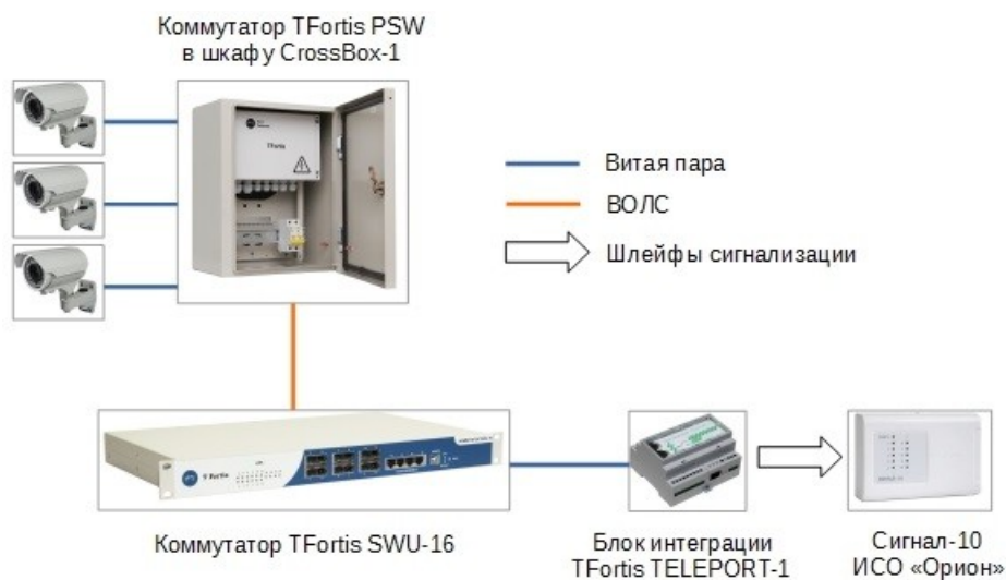
Рис. 5.3.27.1 Структура сети
